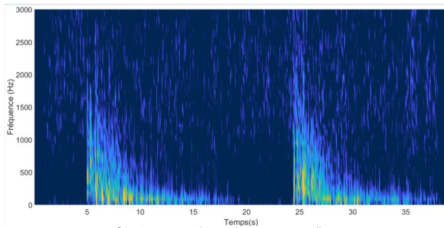
Spectrogramme du son du tonnerre sous l'eau
